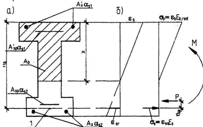
Черт.4.10. Приведенное поперечное сечение (а) и схема напряженно деформированного состояния изгибаемого предварительно напряженного элемента с трещинами (б) при расчете его по деформациям 1 - центр тяжести арматуры растянутой зоны
