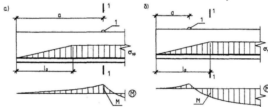
Черт.3.8. К определению момента M при расчете в стадии предварительного обжатия а) - когда a > l_p б) - когда a < l_p ; 1-1 - расчетное сечение; l - монтажная петля
