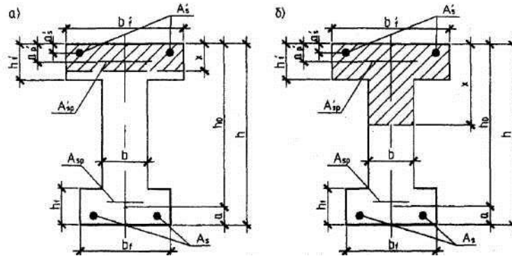
Черт.3.2 Форма сжатой зоны в двугавровом сечении железобетонного элемента а - при расположении границы сжатой зоны в полке; б - то же, в ребре
