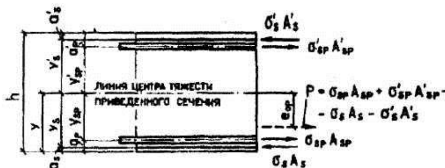
Черт. 2.1 Схема усилий предварительного напряжения арматуры в поперечном сечении железобетонного элемента
