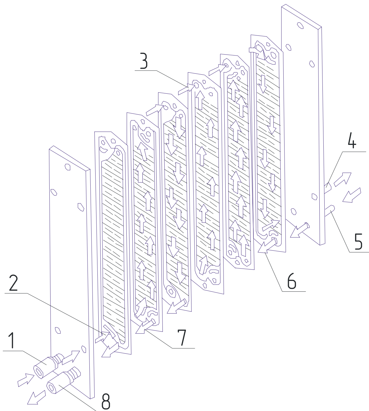
Рис. 1.2 Схема движения теплообменивающих средств в пластинчатом охладителе:
