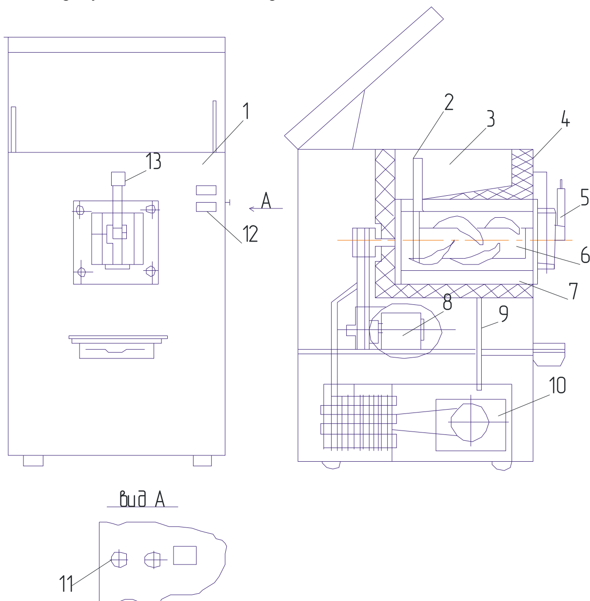
Рис. 8.1 Фризер ФМ-1:
