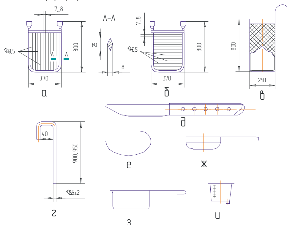
Рис 6.1 Ручной инструмент
