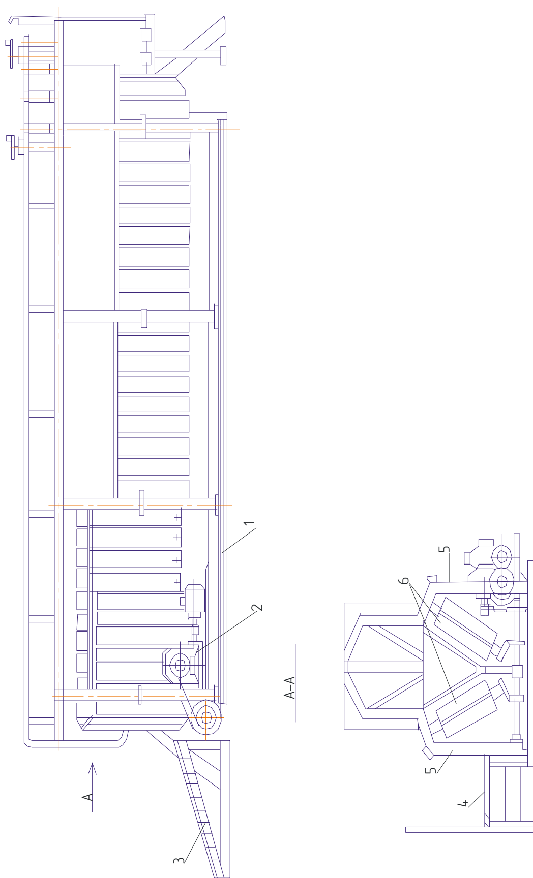
Рис.10.5 Фиксирующий конвейер Г2-ФПКФ для электроглушения свиней:
