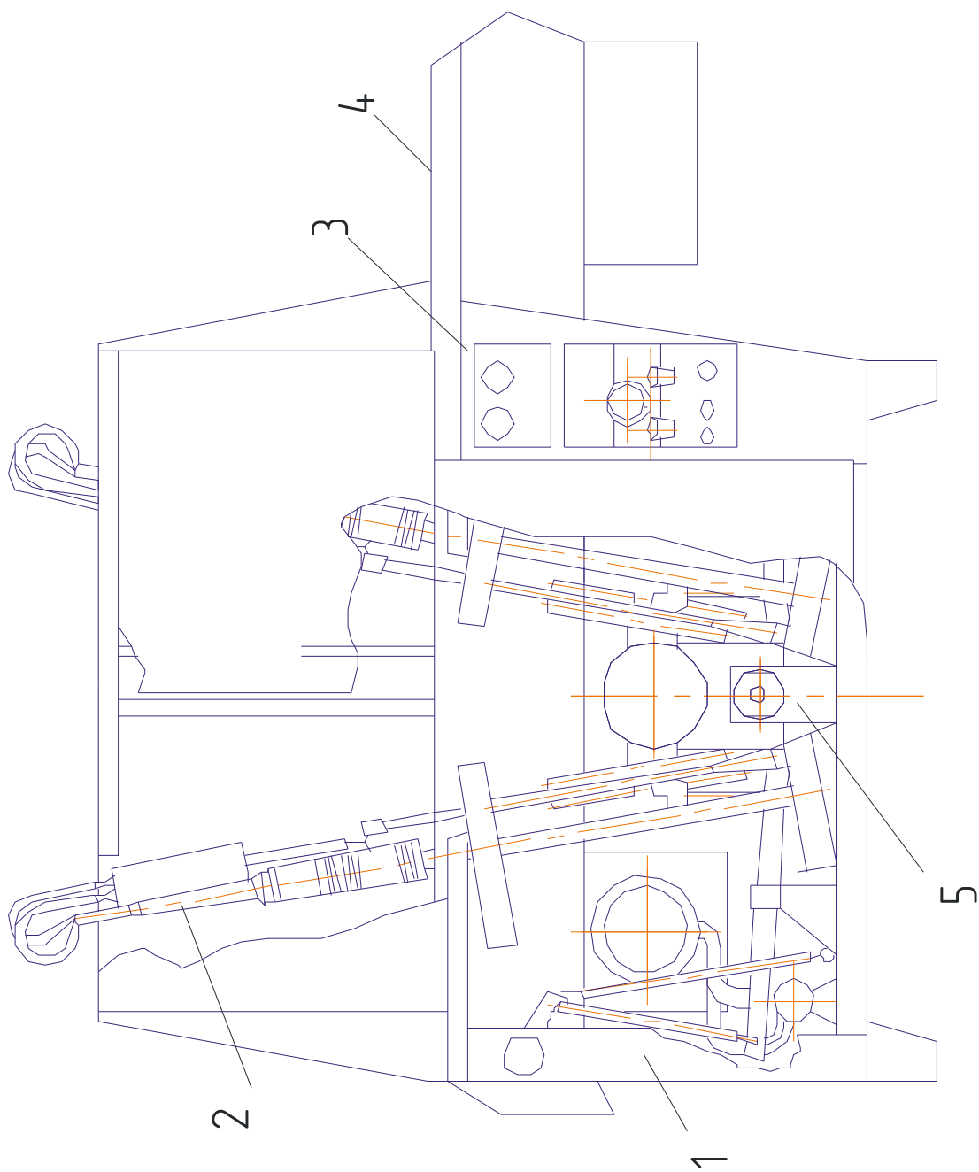
Рис. 12.2 Посолочный автомат ФАП:
