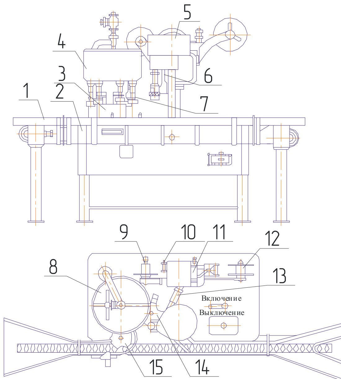
Рис. 9.1 Общий вид фасовочно-укупорочной машины.
