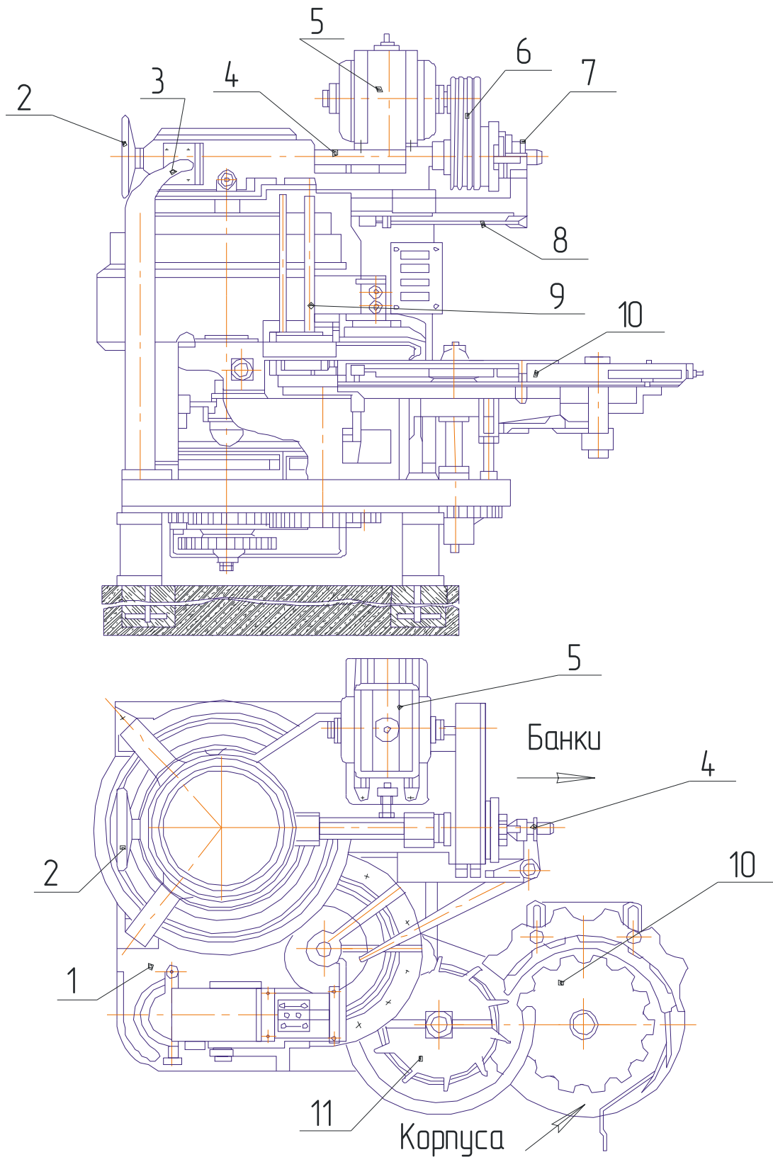
Рис. 15.5 Однобашенная закаточная шестишпindelная машина 1 – станина; 2 – штурвал; 3 – стойка; 4 – вал; 5 – электродвигатель; 6 – клиноременная передача; 7 – муфта; 8 – рукоятка; 9 – магазин для доньшек; 10 – приемная звезда; 11 – разгонная звезда.
