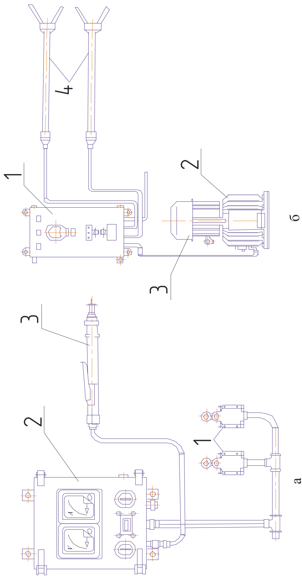
Рис. 10.6. Аппараты для электрооглушения скота:
