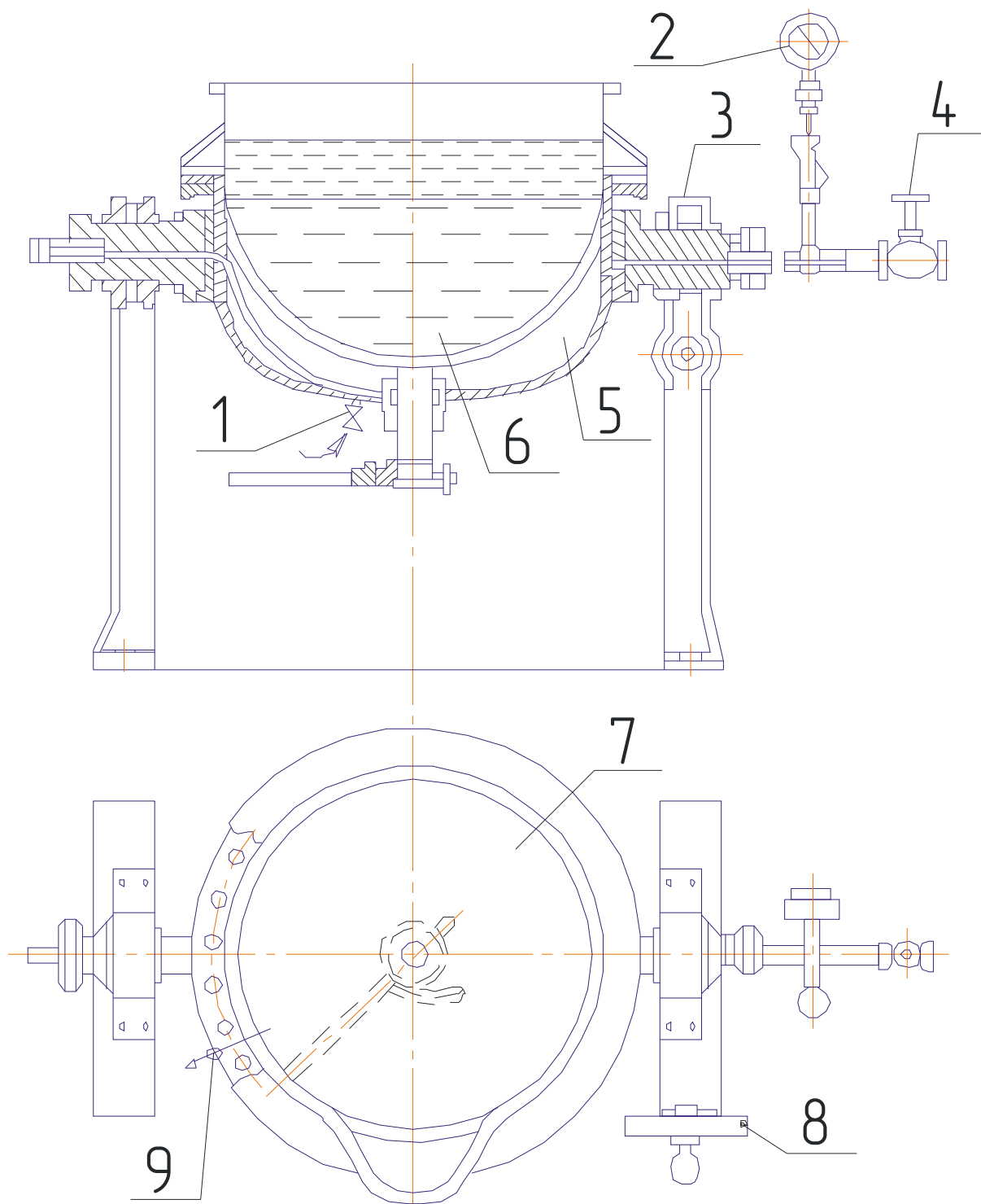
Рис13. 5. Паровой варочный котёл
