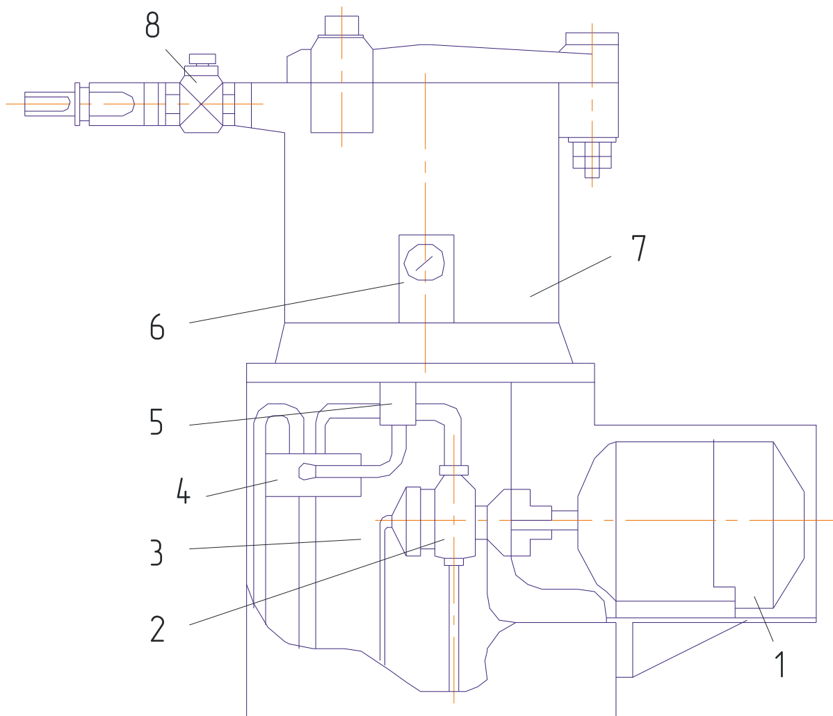
Рис. 14.3 Общий вид гидравлического шприца ГШУ-2:
