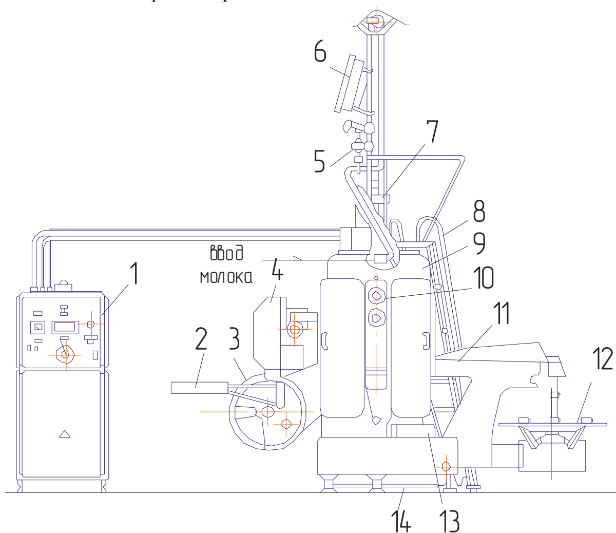
Рис. 9.4 Общий вид автомата фирмы "Тетра Пак"
