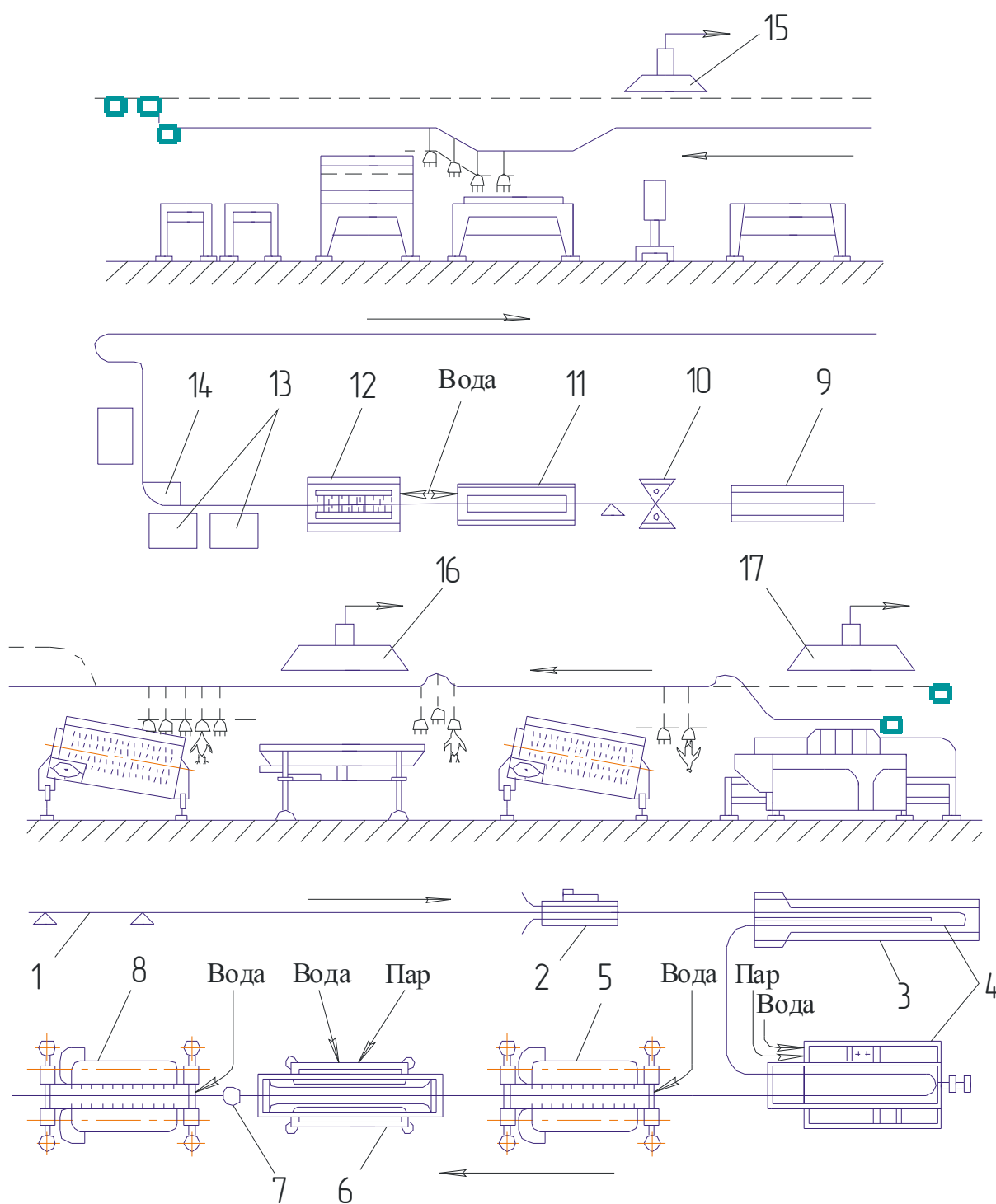
Рис. 10.9. Технологическая схема линии убоя и обработки птицы: 1- подвесной конвейер; 2- аппарат для электрооглушения; 3- лоток для убоя птицы и сбора крови; 4- аппарат для тепловой обработки; 5,8- бильные машины; 6- аппарат подшпарки; 7- точка подвеса; 9- лоток ручной дооципки; 10- камера газовой опалки; 11- стол полупотрошения; 12- камера мойки; 13- столы сортирования, маркирования и упаковывания; 14- натяжная станция; 15,16,17- вытяжные зонты.
