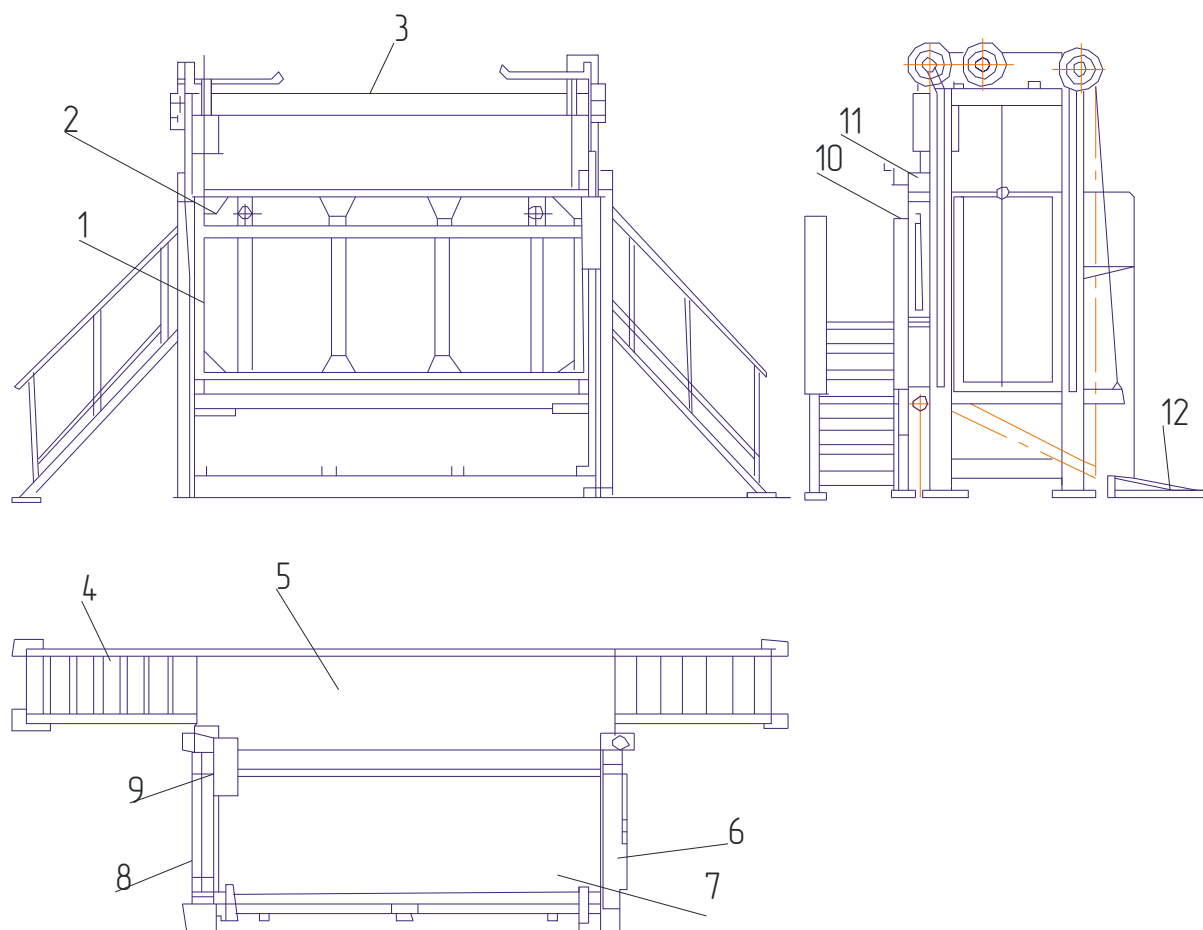
Рис. 10.3 Бокс Г6-ФБА для оглушения крупного рогатого скота:
