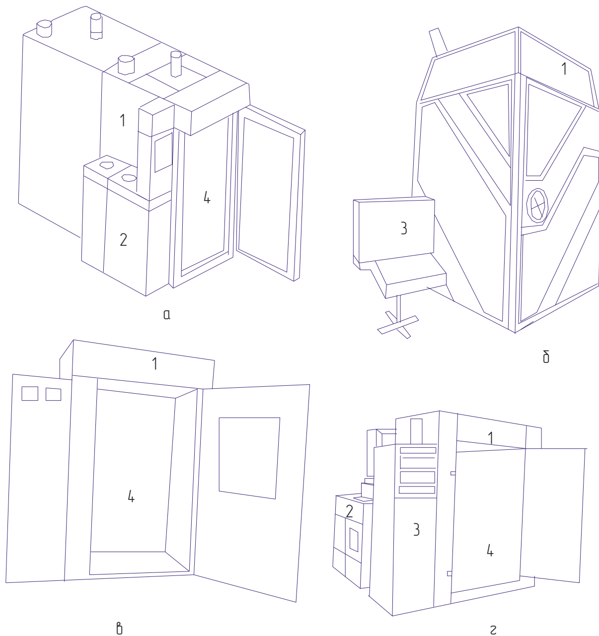
Рис. 13.4. Универсальные термокамеры:
