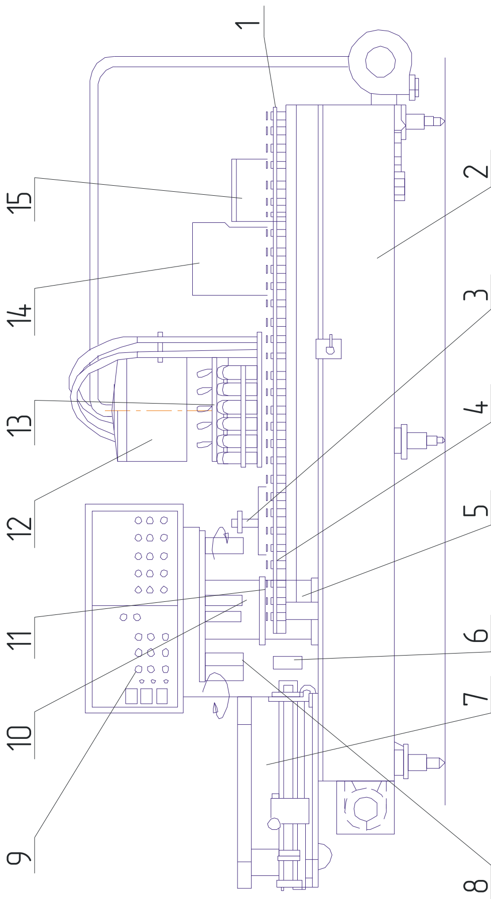
Рис. 9.6 Фасовочно-упаковочный автомат системы "Пюр Пак":
