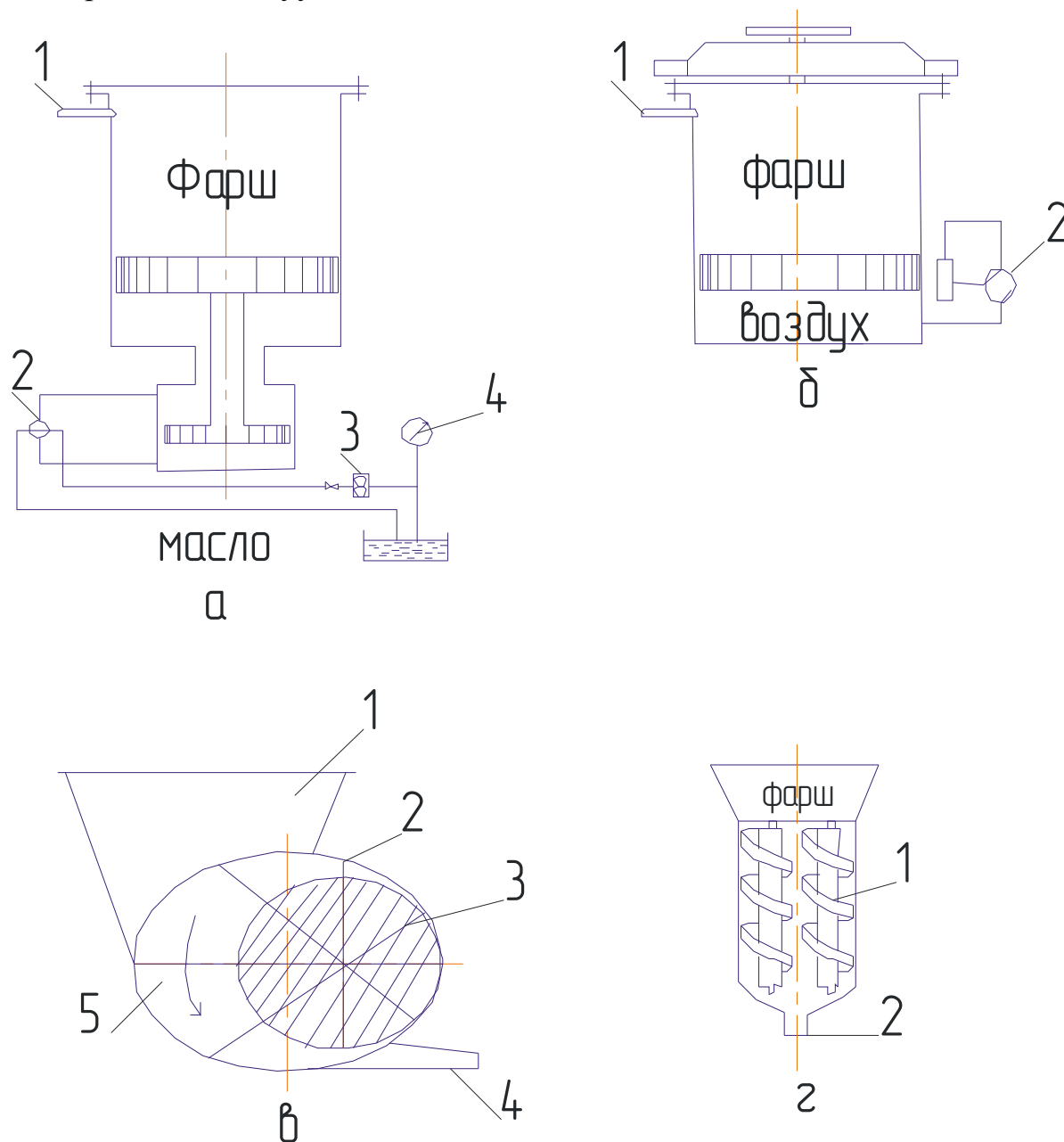
Рис. 14.1. Схема работы шприцев:
