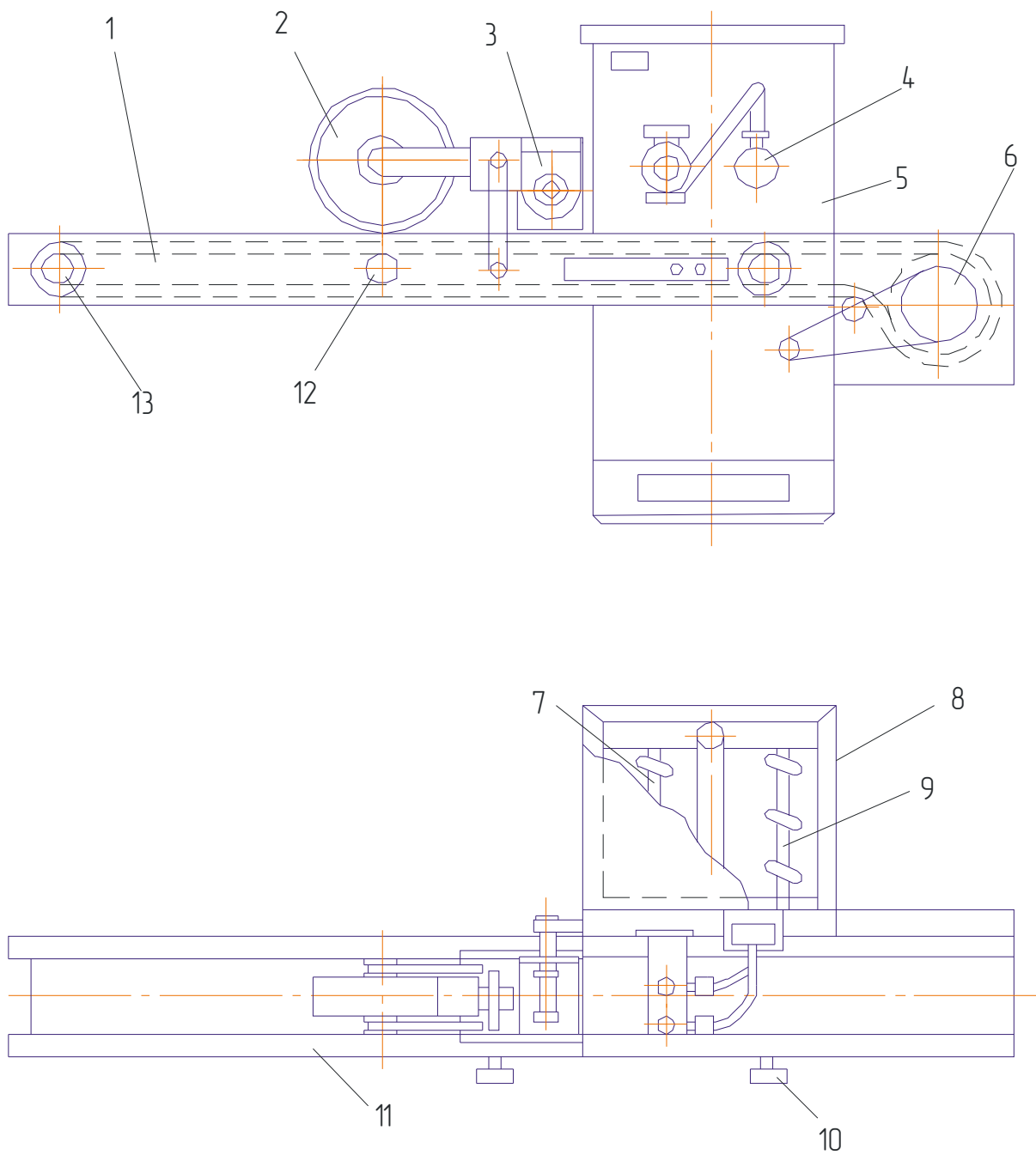
Рис 14.8 Пельменный автомат СУБ-2-67:
