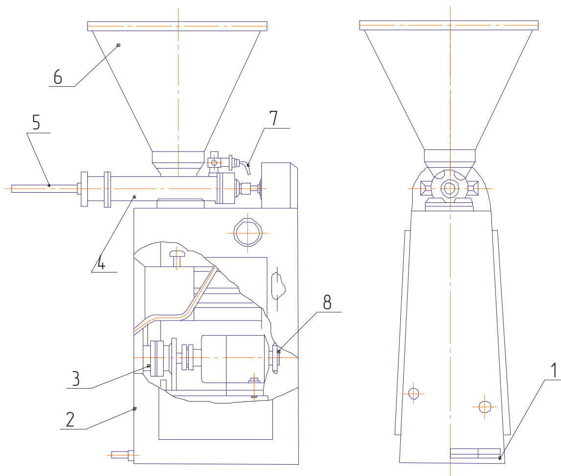
Рис. 14.4. Двухцветочный вакуумный шприц ФШ2-ЛМ:
