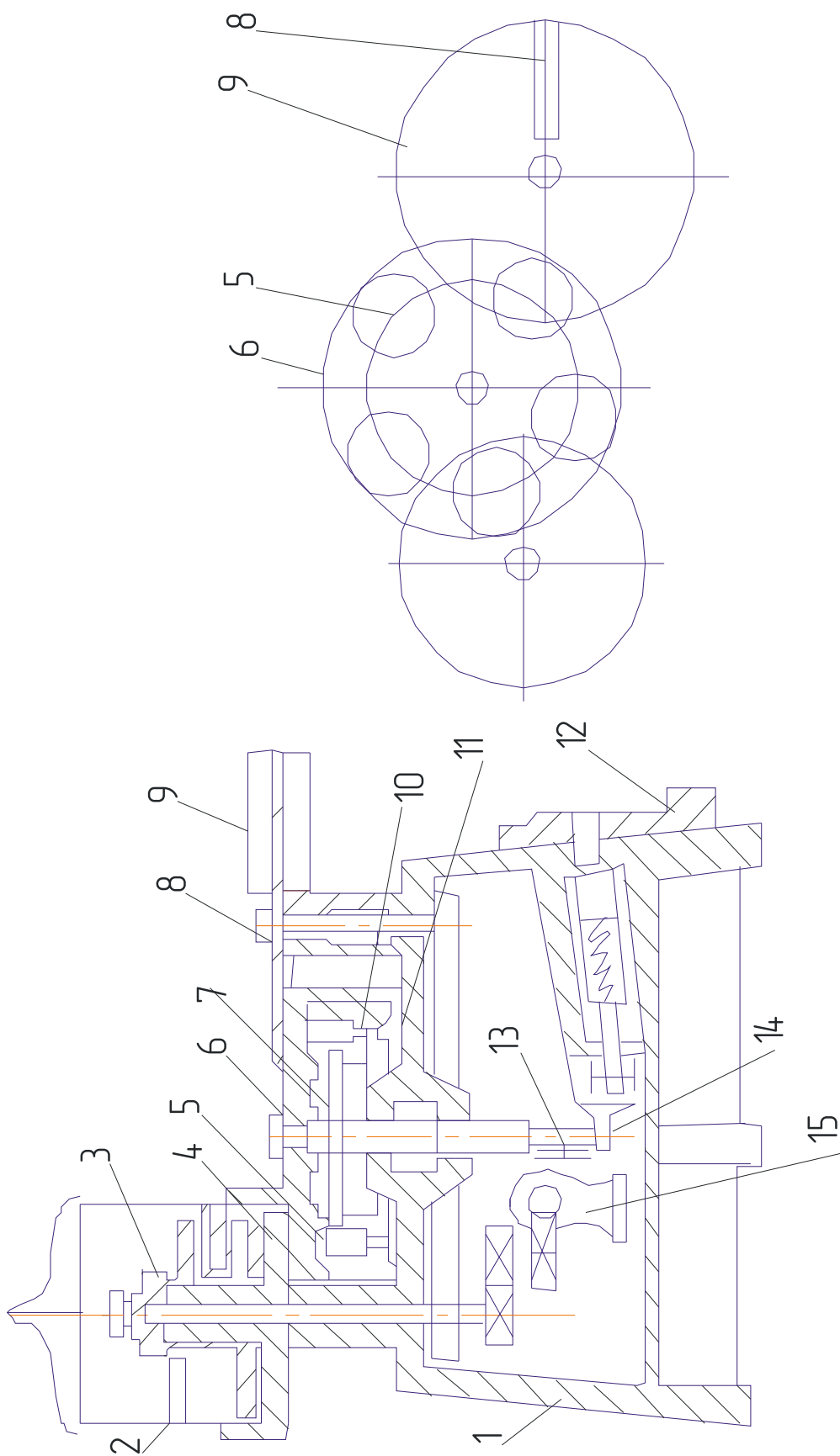
Рис. 14.6. Котлетный автомат АК2М-40:
