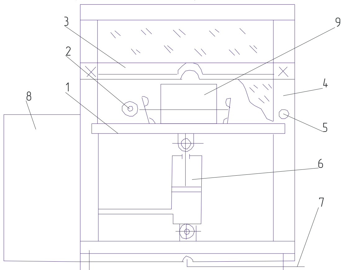
Рис. 11.3. Схема машины Г6-ФРА:
