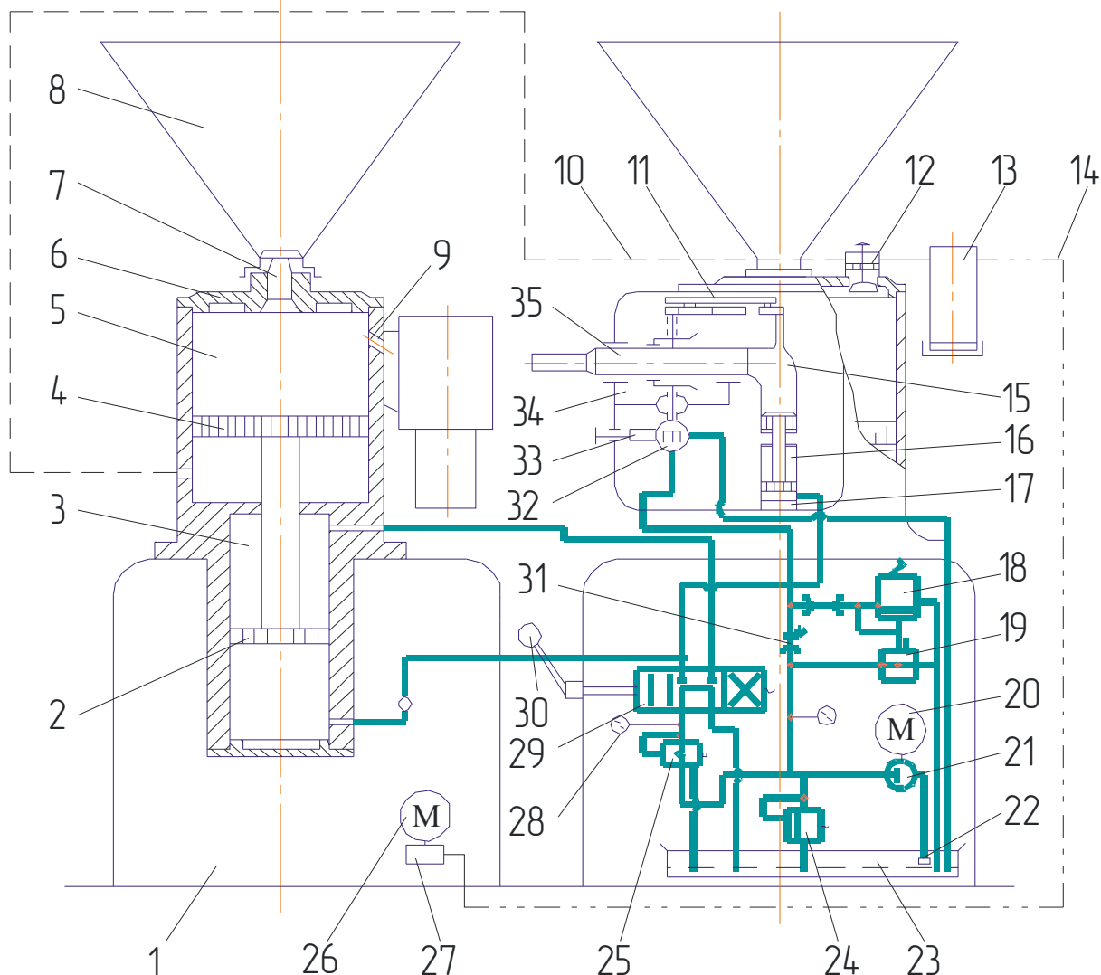
Рис. 14.2 Комбинированная схема гидравлического шприца-дозировщика Е8-ФНА-01:
