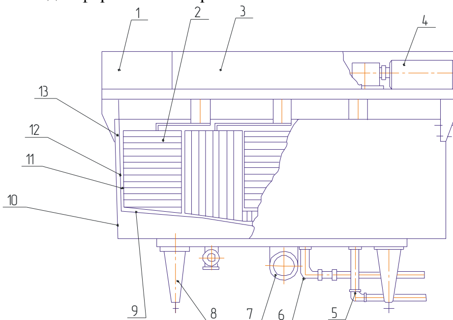
Рис. 6.2 Сыроизготовитель Я5 - ОСЖ - 1:
