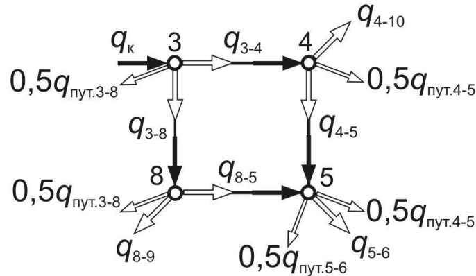
Рисунок 3 — Распределение воды в кольце
