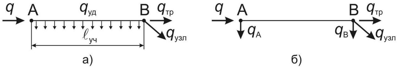
Рисунок 1 — Замена равномерного путевого расхода сосредоточенным: а) — участок сети до замены; б) — участок сети после замены
