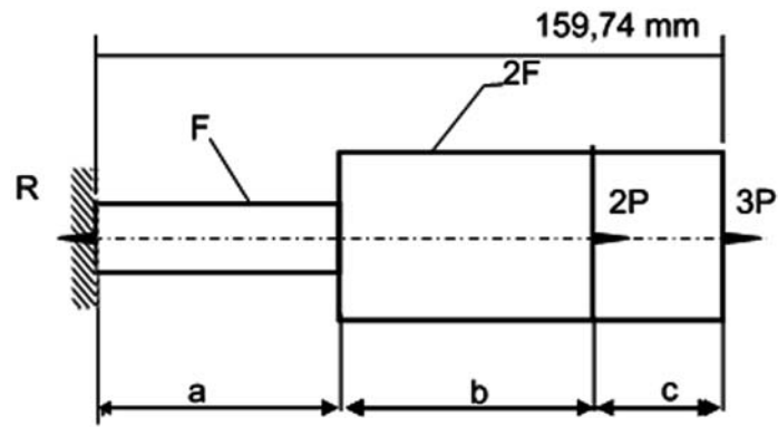
Рис. 2.14. Схема конструкции
