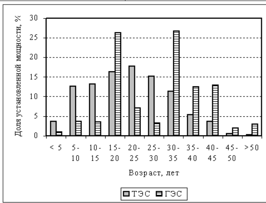
Рис. 3. Возраст ТЭС и ГЭС РАО «ЕЭС России» на конец 1998 г.
