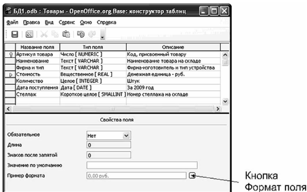
Рис. 3. Заполнение структуры таблицы
