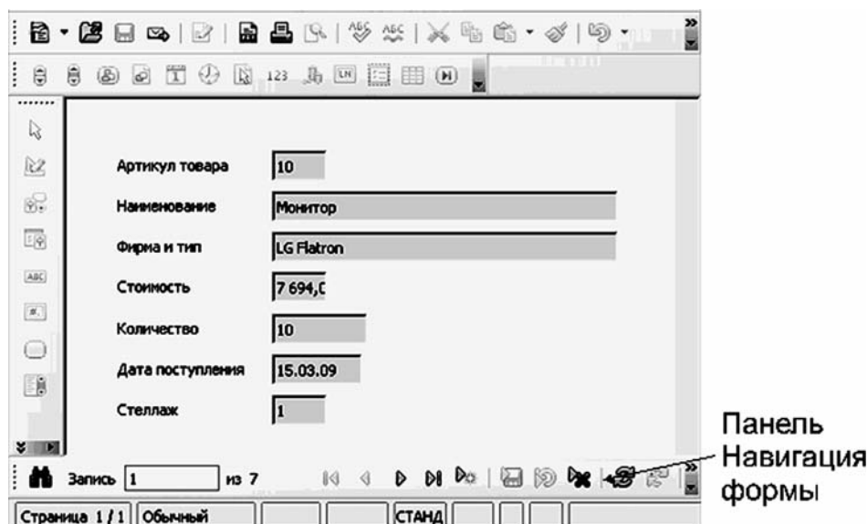
Рис. 4. Форма для созданной таблицы
