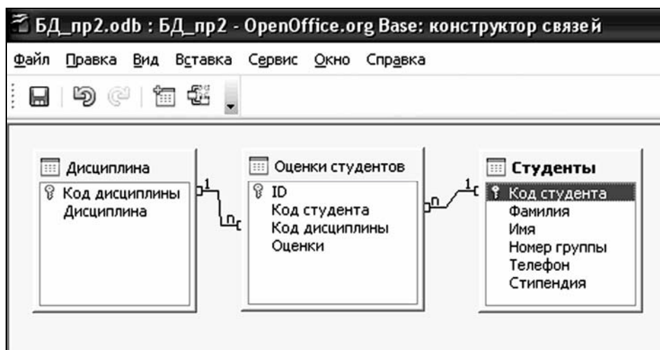
Рис. 11. Макет связи между таблицами БД Деканат
